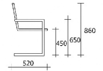
Grundmaße in mm
